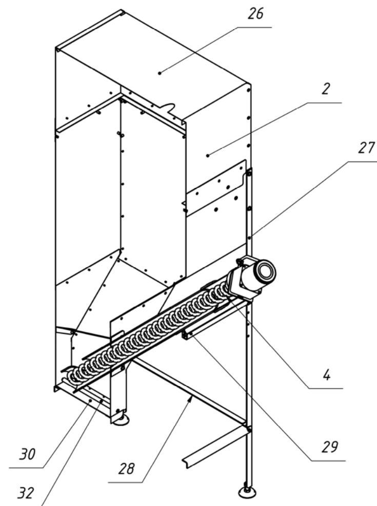
Рис. 3б Бункер с податчиком пеллет.
